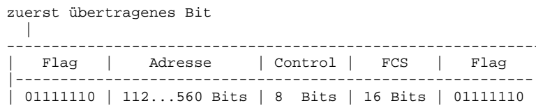
Abb. 1A - Aufbau von U und S Blocks
