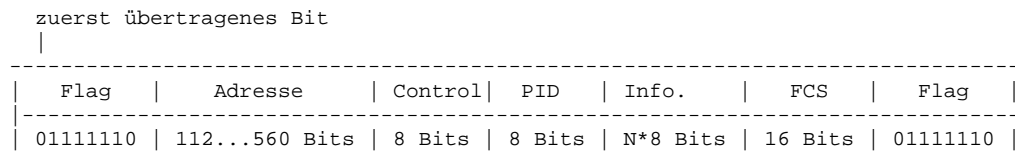
Abb. 1B - Aufbau von Informationsblocks
