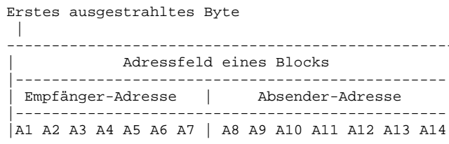
Abb. 2 -- Kodierung des Adressfeldes ohne Digipeater
