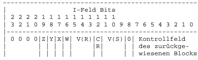
Abb. 7 -- I-Feld des FRMR-Blocks
